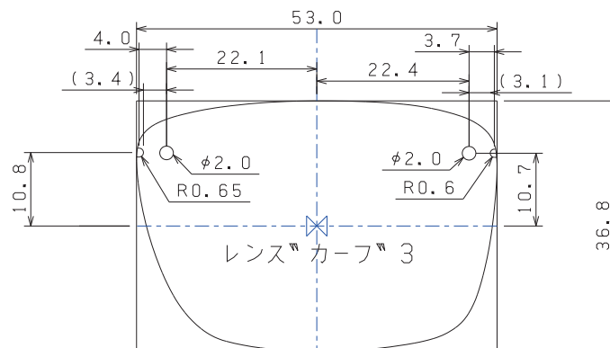
レンズ ㊦ 形状
