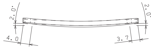
レンズ ㊦ 形状
